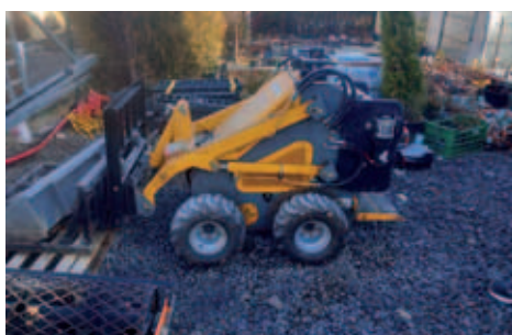
Hydraulický manipulátor M. Štencla
